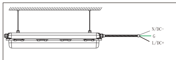
Pendant Mount
